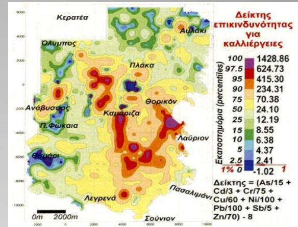
Σχήμα 16. Γεωχημικός χάρτης κατανομής του Δείκτη Επικινδυνότητας για καλλιέργειες στη Λαυρεωτική χερσόνησο ως προς τα τοξικά χημικά στοιχεία αρσενικού (As), καδμίου (Cd), χρωμίου (Cr), χαλκού (Cu), νικελίου (Ni), μολύβδου (Pb), αντιμονίου (Sb) και ψευδαργύρου (Zn). Η λευκή οδοντωτή γραμμή δείχνει το όριο που θεωρείται ασφαλές για καλλιέργειες, που είναι μόνο το 1% της έκτασης της Λαυρεωτικής χερσονήσου.
